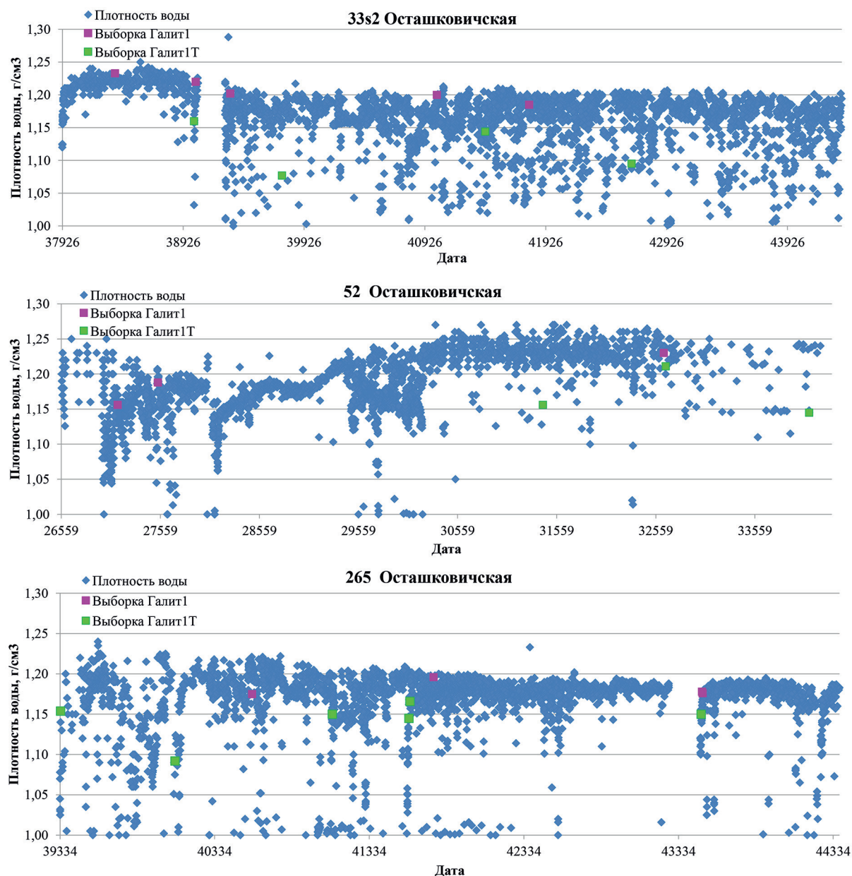
Рисунок 1 – Изменение плотности попутных вод по скв. 33s2, 52, 265 Осташковичского месторождения
