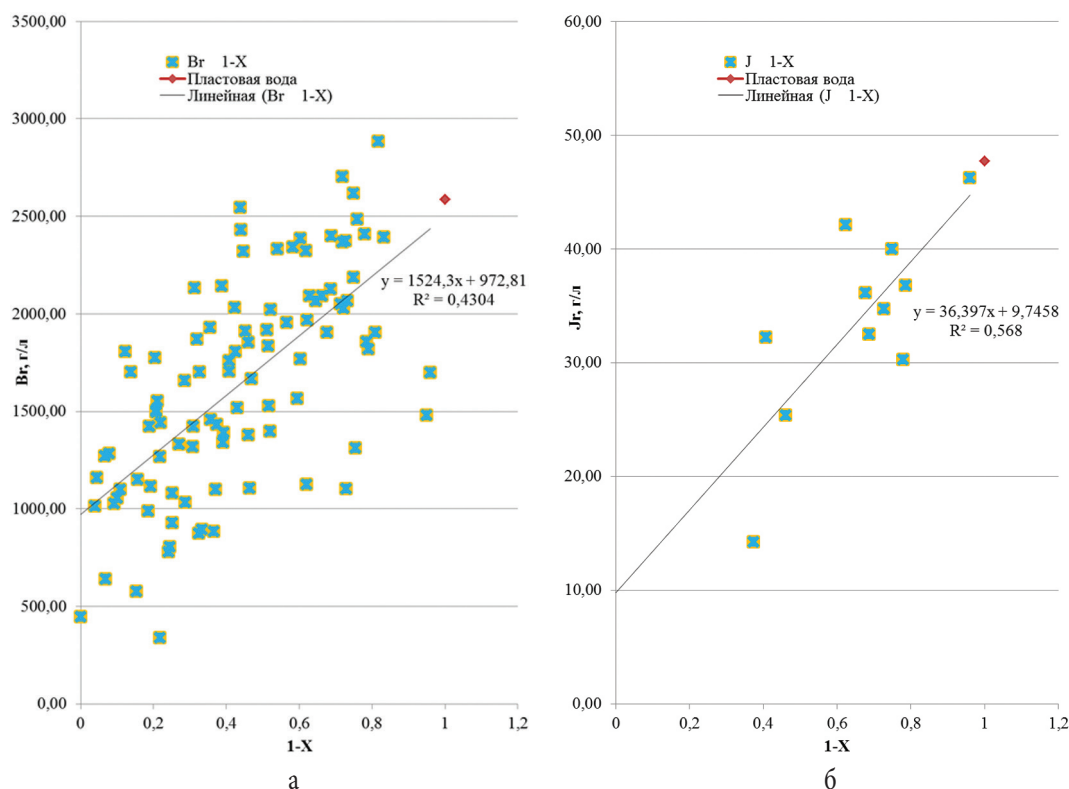
Рисунок 3 – Зависимость осредненных по скважинам концентраций брома (а) и йода (б) в попутных водах межслоевой залежи нефти Осташковичского месторождения от долевого участия в них пластовых рассолов
